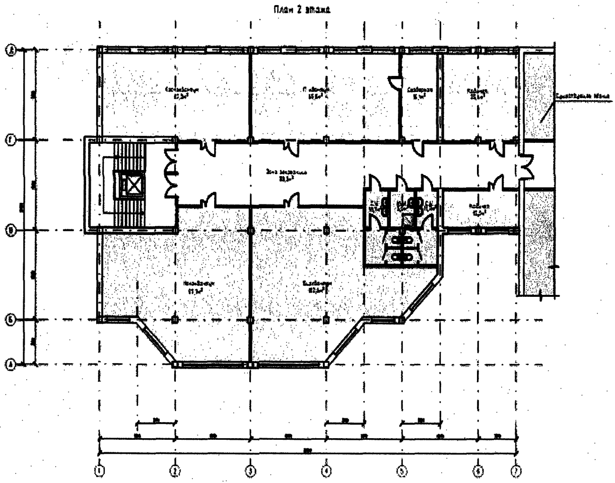
Рисунок 2. План зонирования помещений 2 этажа
