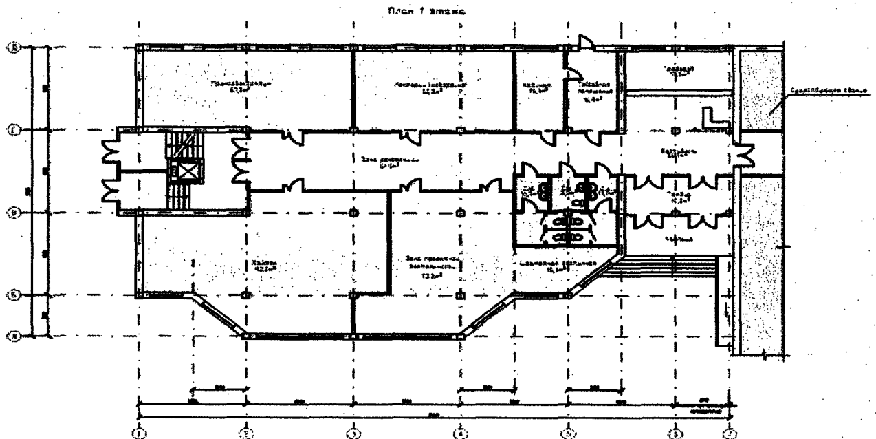
Рисунок 1. План зонирования помещений 1 этажа
